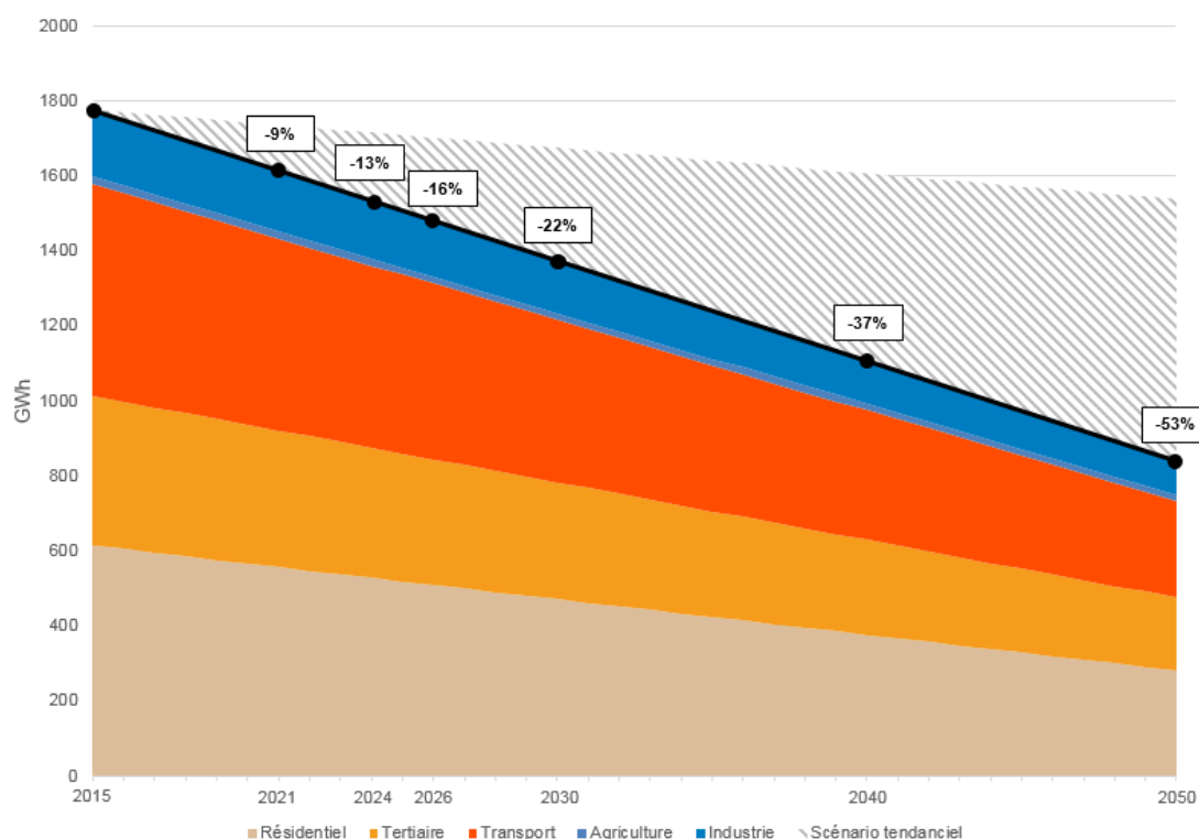
Figure 12. Trajectoire CAVBS des consommations énergétiques en comparaison avec la trajectoire tendancielle (Source : Algoé)
