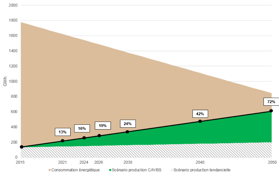
Figure 15. Part de la production énergétique (volontariste et tendancielle) au regard de la réduction des consommations énergétiques (Source : Algoé)
