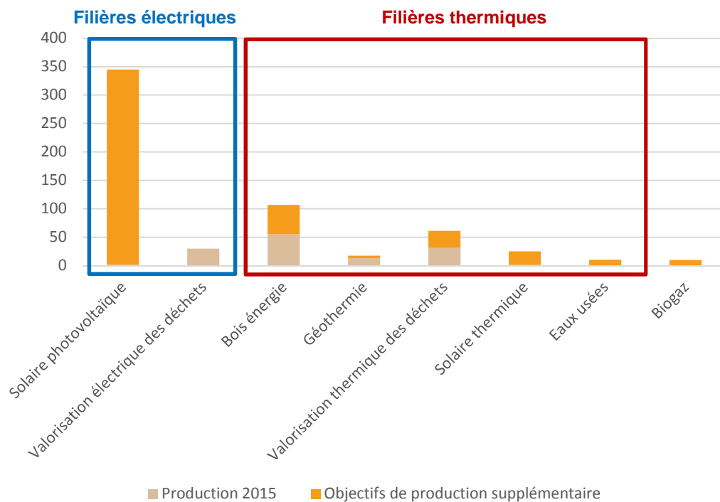
Figure 14. Objectifs de production d'énergie renouvelable mobilisable à l'échelle du territoire de la CAVBS (Source : Algoé)
