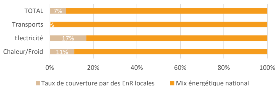
Figure 16. Part des énergies renouvelables et de récupération dans le mix énergétique global pour l'année de référence 2015 (Source : Algoé)
