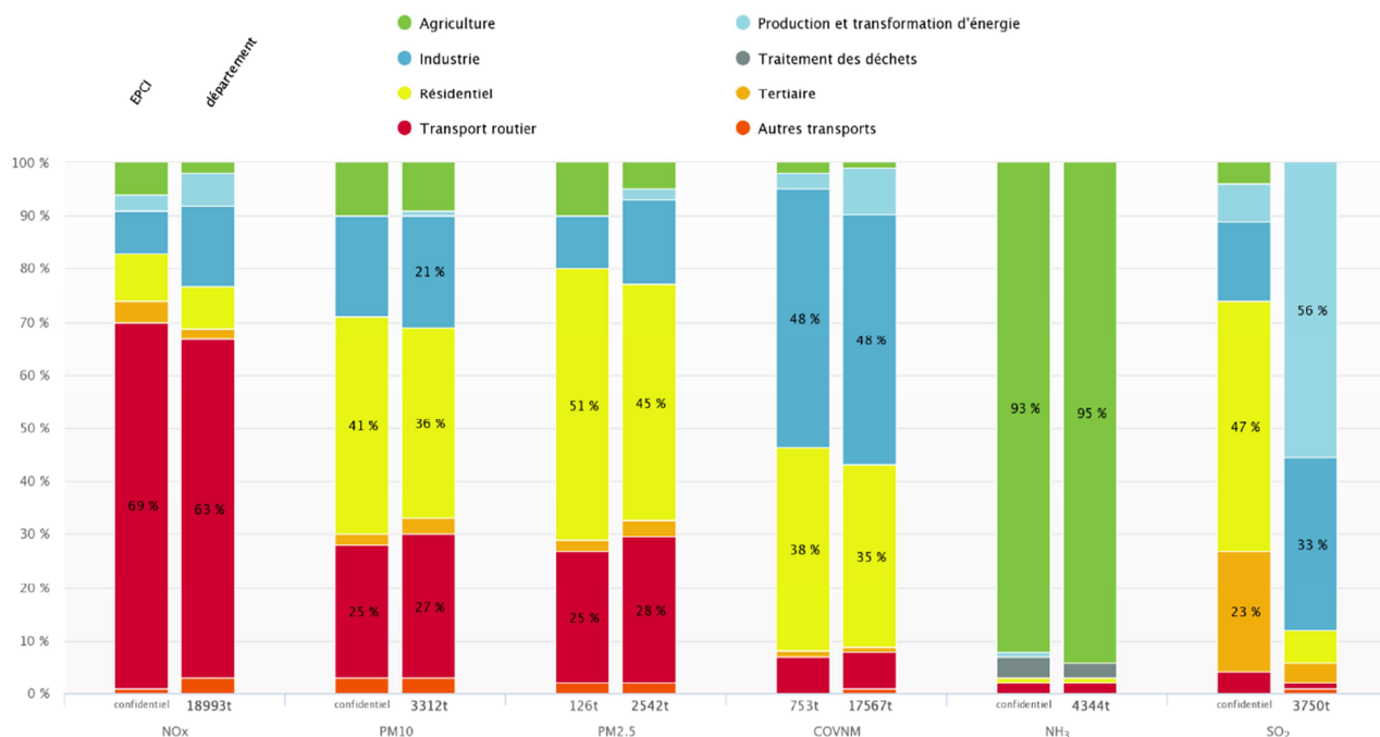
Figure 5. Consommation d'énergie par besoin et par secteur en 2016 Source : ©Atmo Auvergne - Rhône-Alpes (2017) Observatoire Fiche territoriale CA Villefranche Beaujolais Saône
