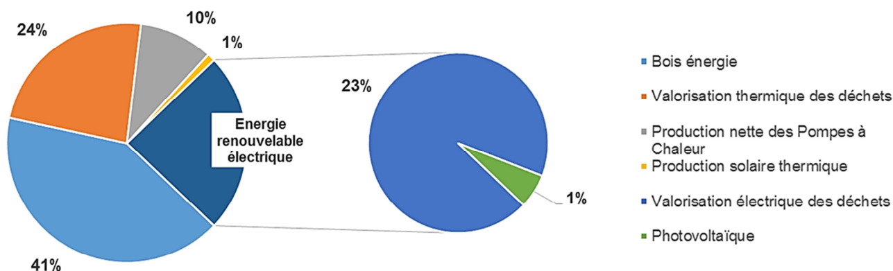
Figure 6. Production d'énergie renouvelable et de récupération par filière (à gauche, chaleur ; à droite, électricité) estimée pour l'année 2015 Source : BG d'après OREGES
